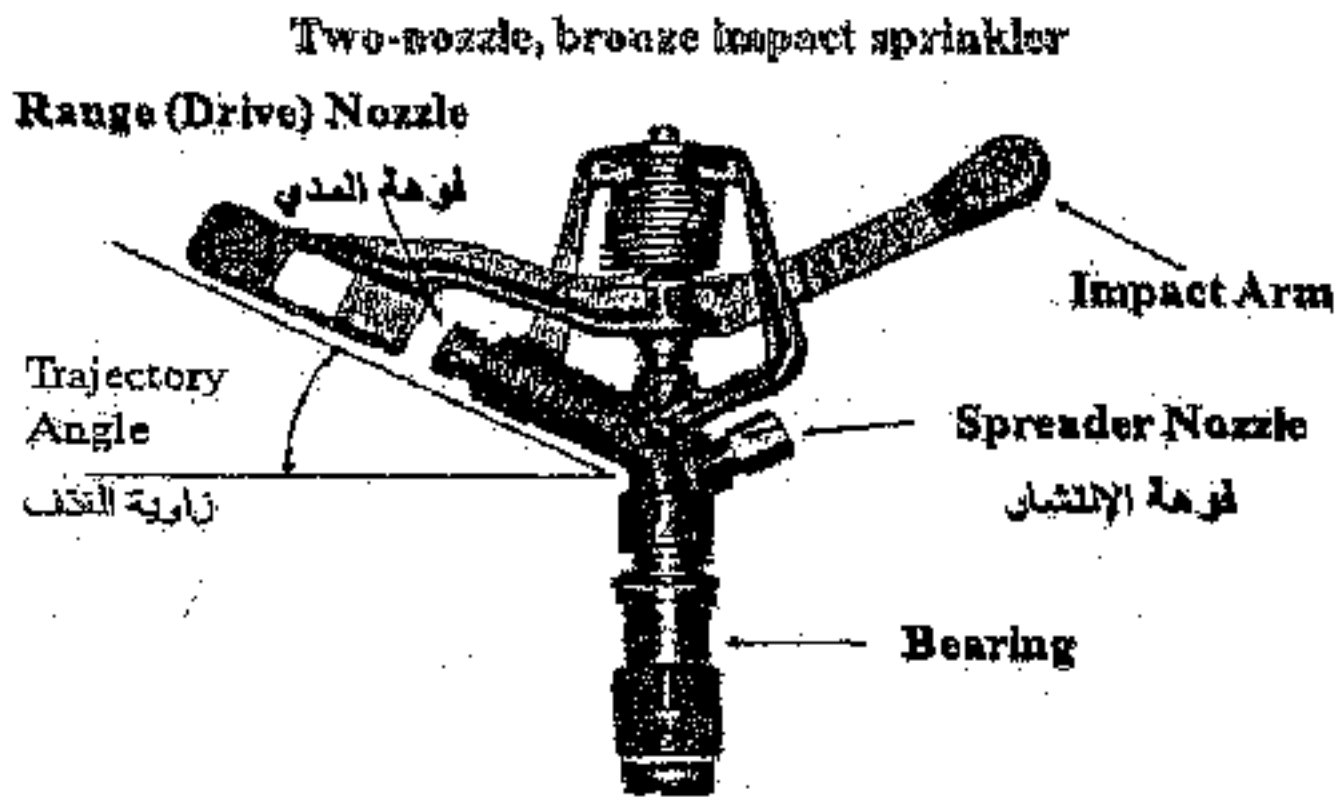
شكل ( ١ ) تركيب الرشاش الدوار
