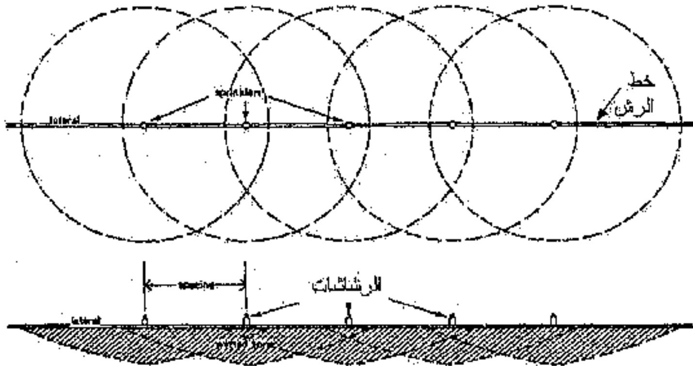
قد لخل دو قطر الرش للرشاشات للخصول على توزيع مياه منتظم
