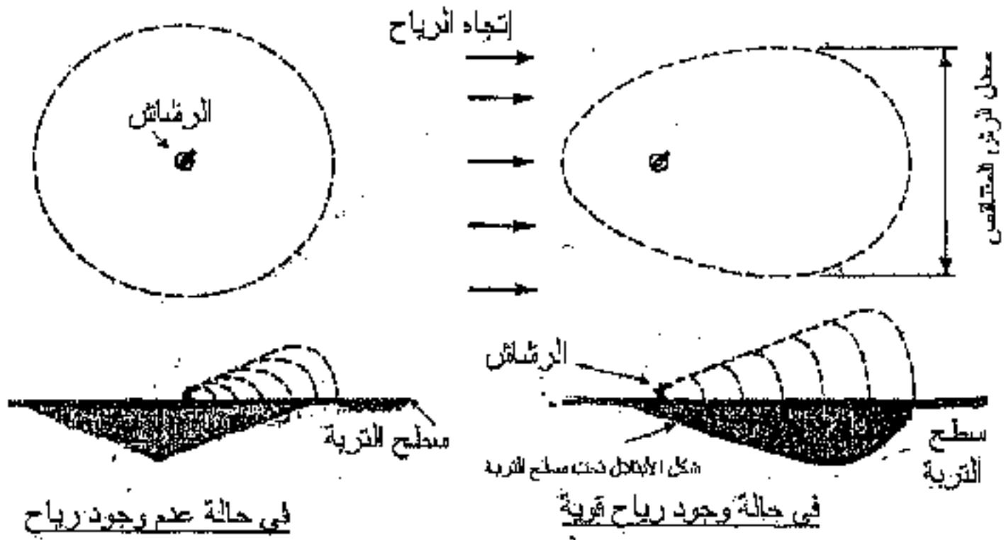
تأثير رياح على توزيع المياه الخارجة من الرشاش
