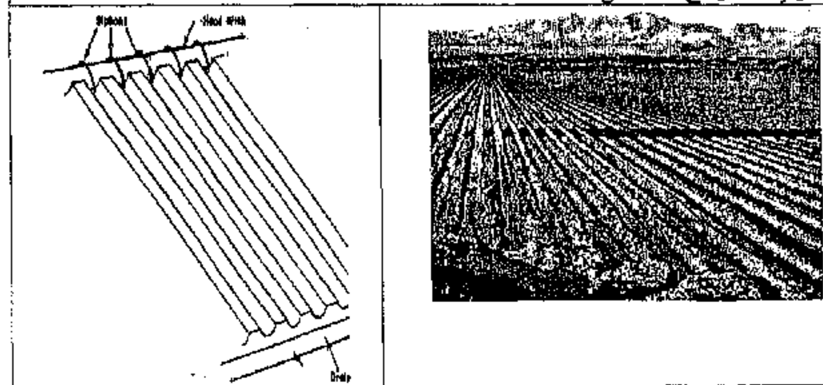
الري بالخطوط Furrow Irrigation
