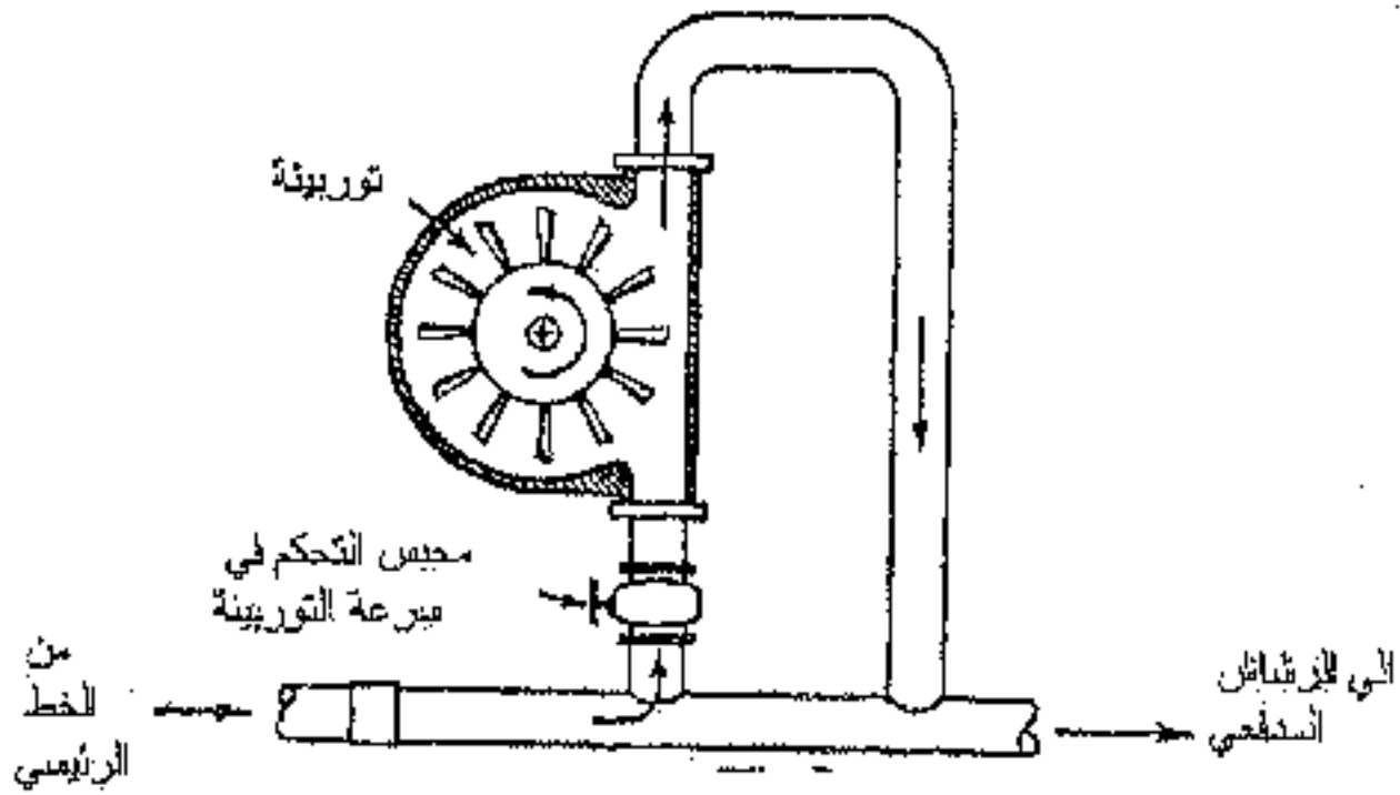
توربينة لدارة الرشاش المدفعي المتحرك
