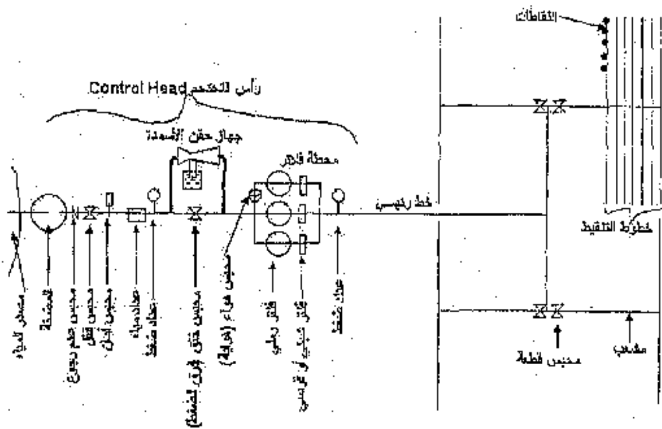
مكونات شبكة الري بالتلقيح
