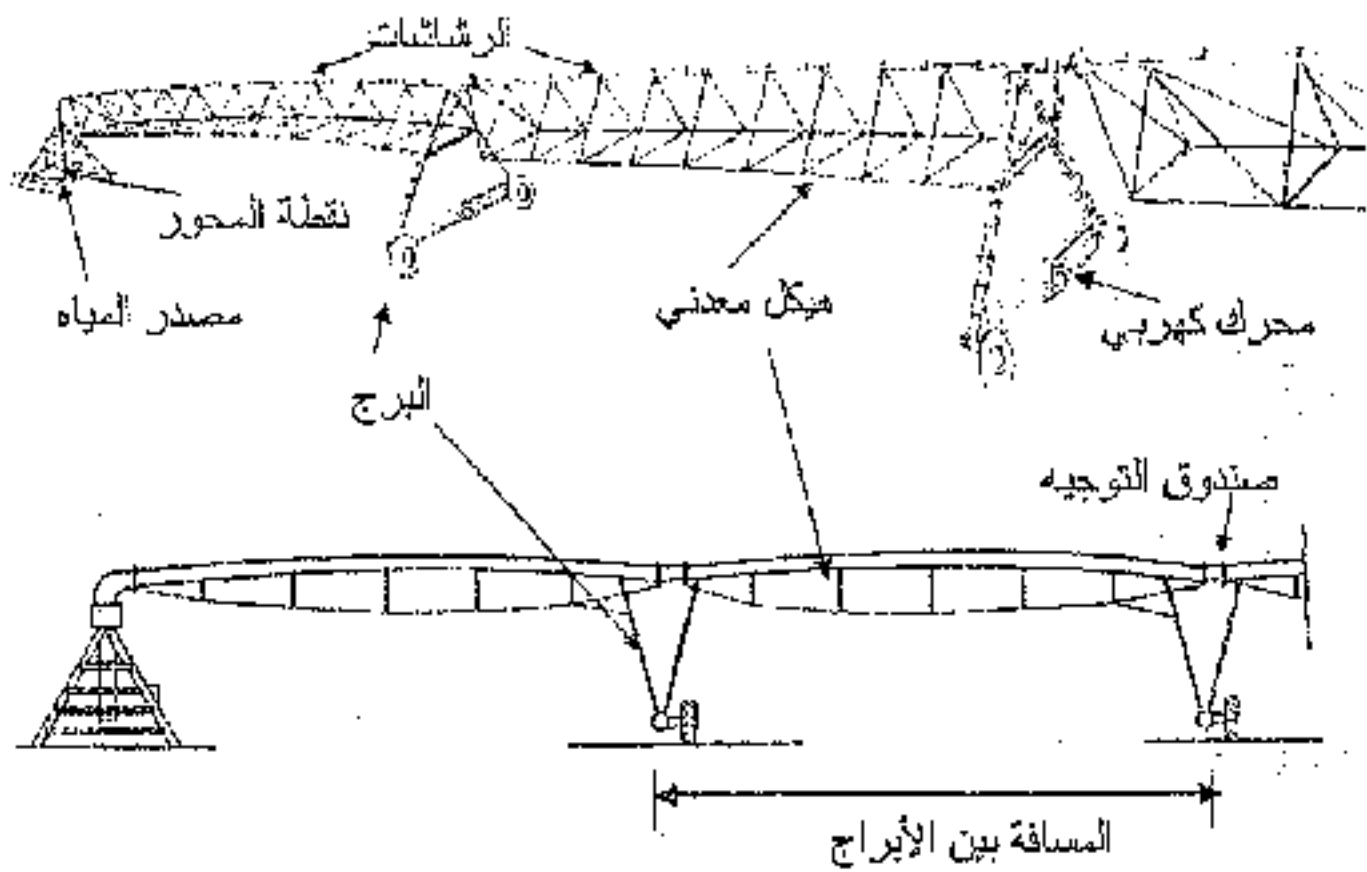
الأجزاء الرئيسية لجهاز الري بالرش المحوري
