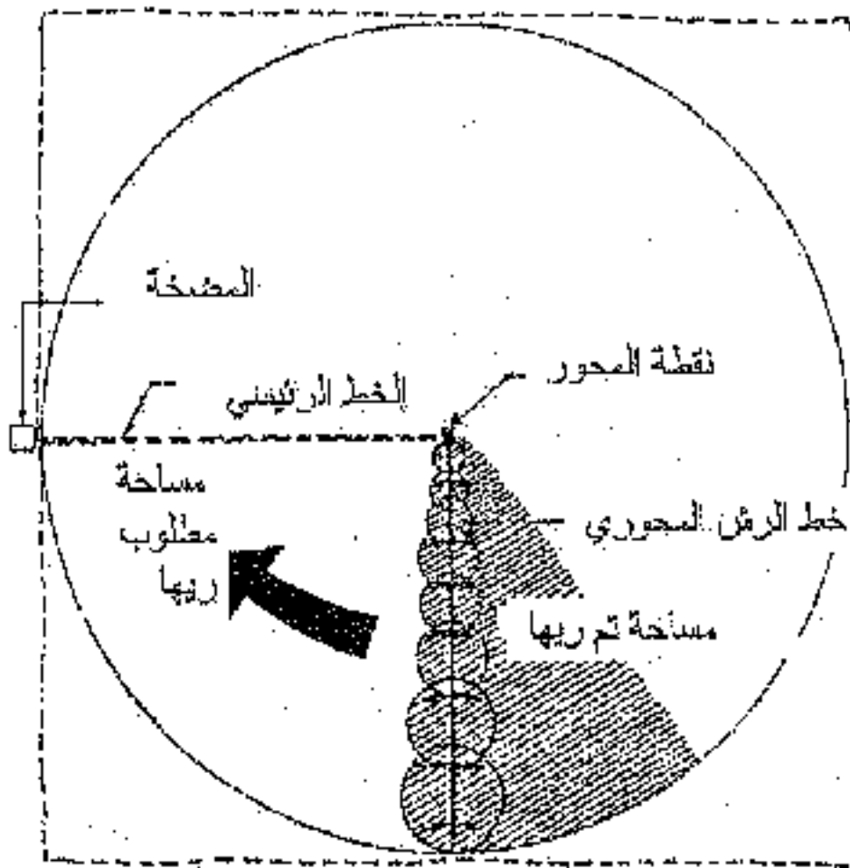
تخطيط حقل نمطي يروي بالري المحوري
