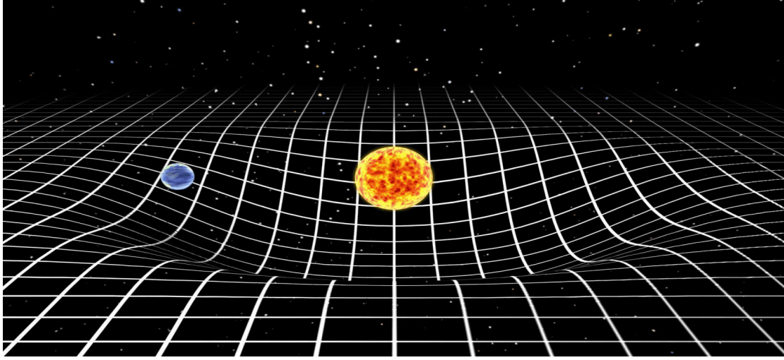
صورة توضيحية لتسيج الزمكان
